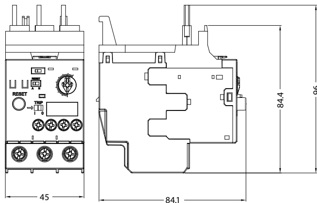
WRB40E
